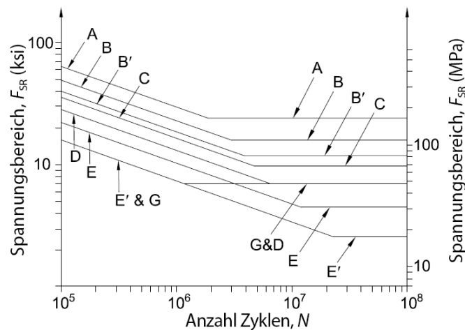
Abb. C-A-3.1 Ermüdungsbeständigkeitskurven.
