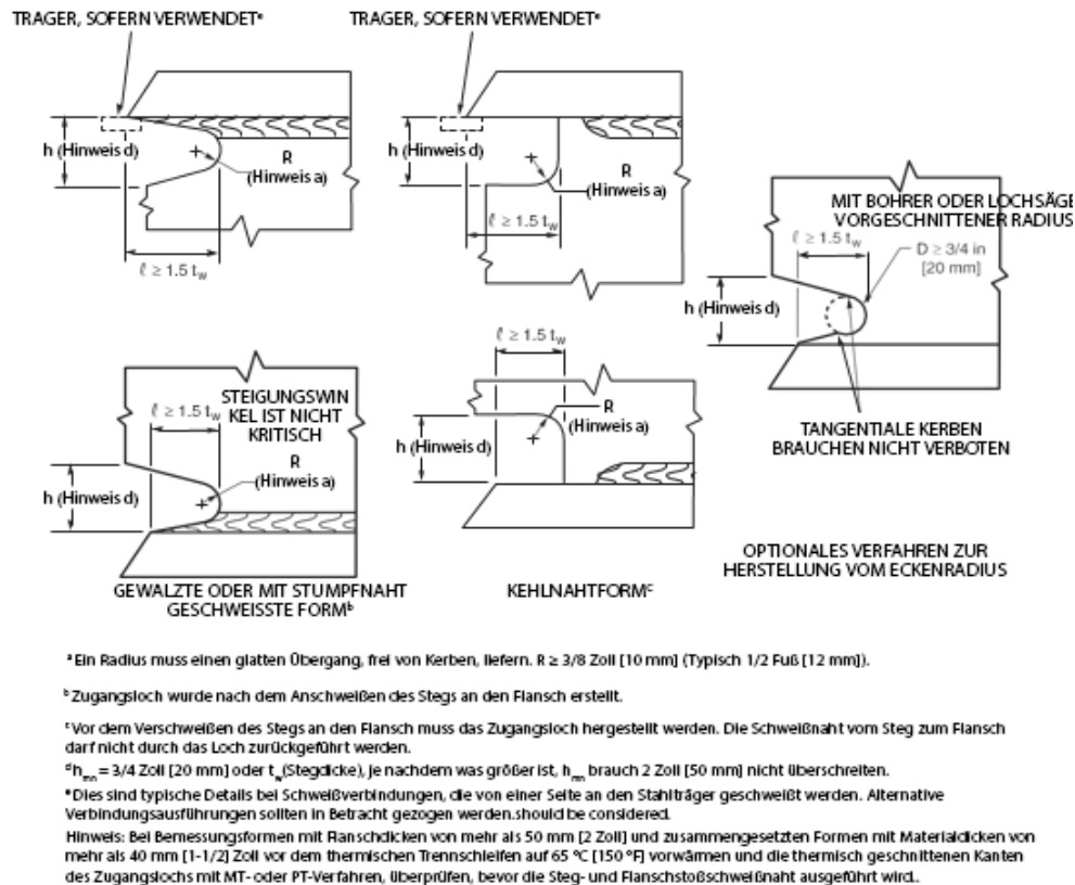
Abbildung 5.2 - Geometrie der Schweißnahtzugangs Löcher (siehe 5.16.1.2)
