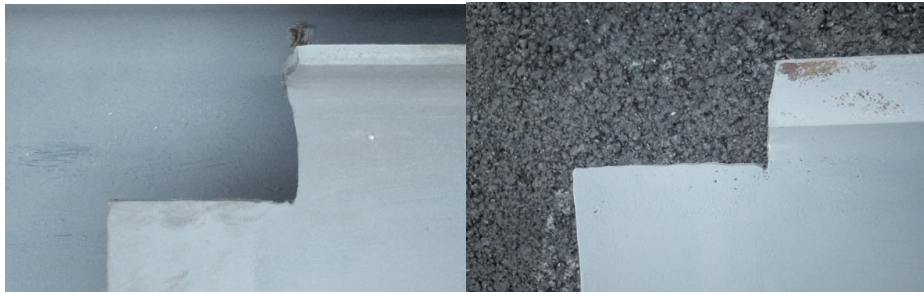
Abbildung 6. Schlechte Praktiken beim Schneiden von Trägersauklinkungen
