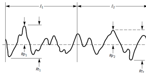
Abbildung 22. ASME B46.1, Abbildung 1-10, Oberflächenprofilmessung
